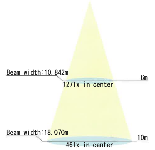
90° レンズ
