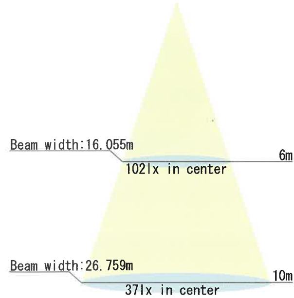
120° レンズ
