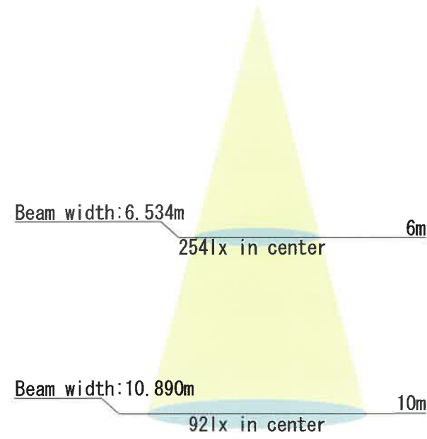
70° レンズ
