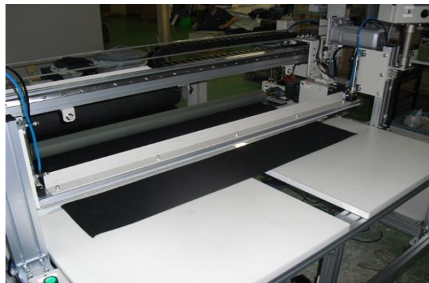
取り除き作動式裁断装置 OSC-1100
